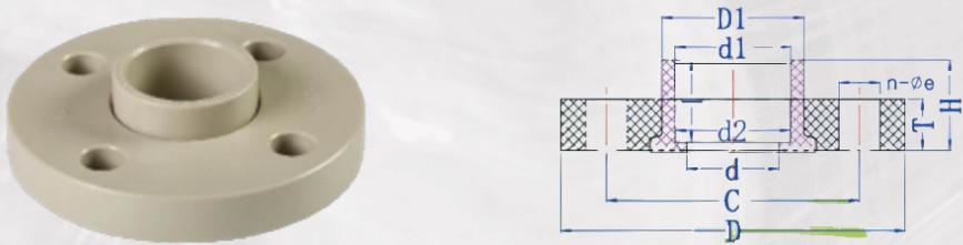
双片法兰 VAN STONE FLANGE
