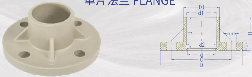
单片法兰 FLANGE
