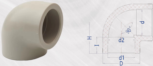
90°弯头 90°ELBOW弯头
